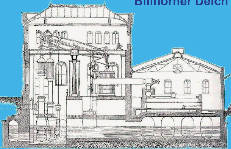
Hamburger Wasserwerk mit Cornwall-Pumpen
