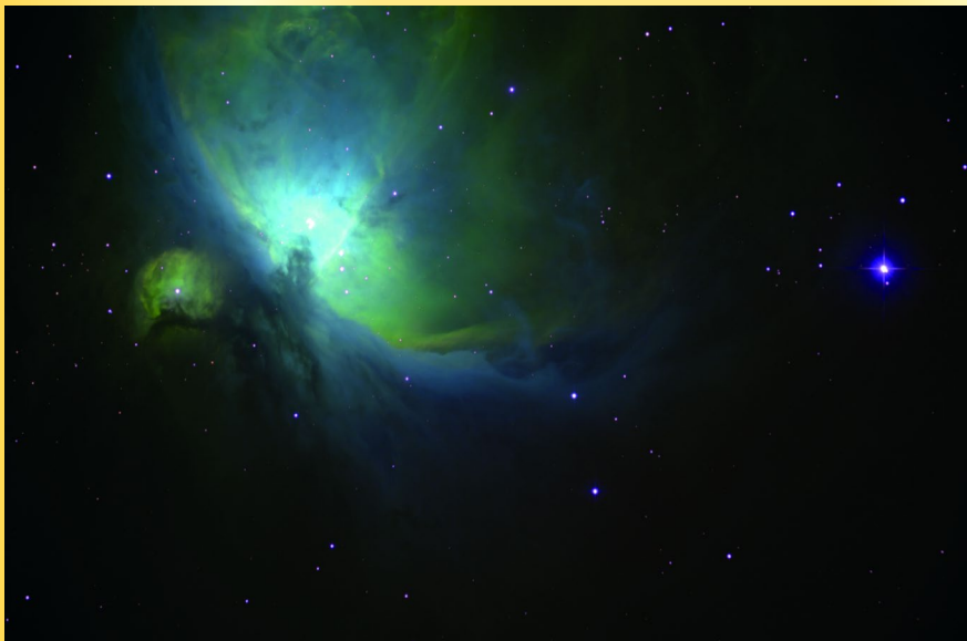
Orionnebel – Ort der Stern- entstehung
