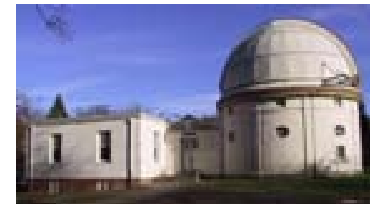
1-M-Spiegelteleskop
