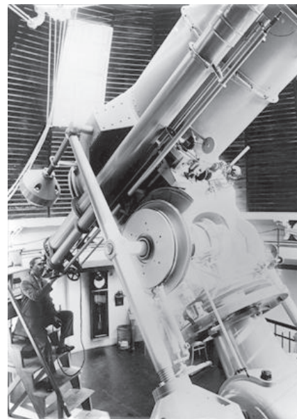
Dr. Walter Baade (1893-1960) am 1m-Spiegel (© Hamburger Sternwarte)
