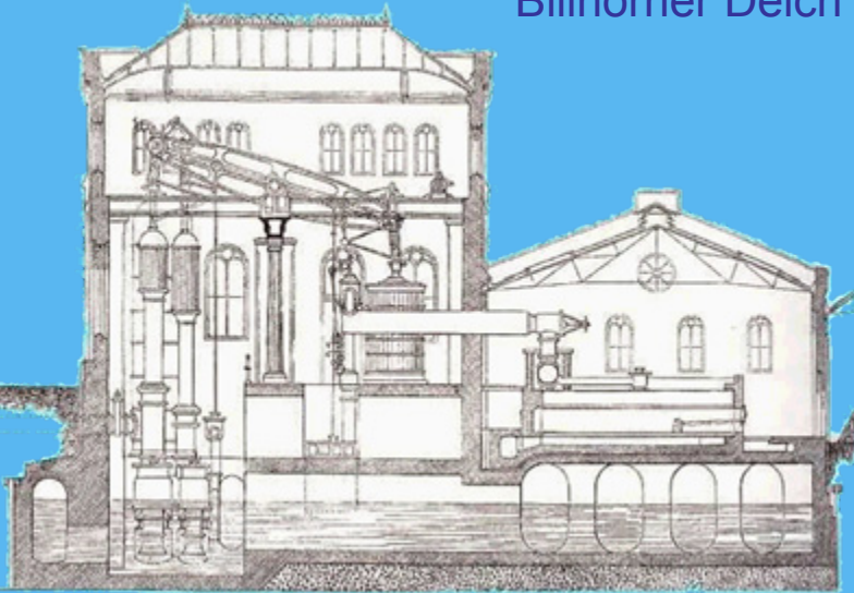
Hamburger Wasserwerk mit Cornwall-Pumpen
